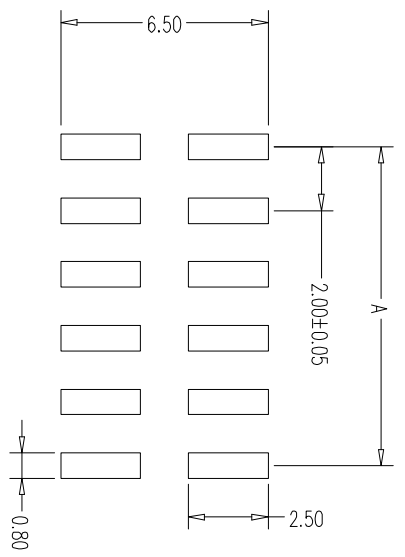
P.C.B Layout
